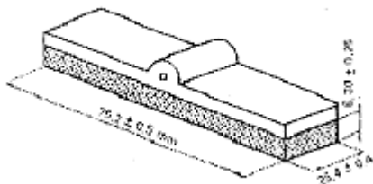
Hình 4 - Tấm trượt gắn đế cao su
