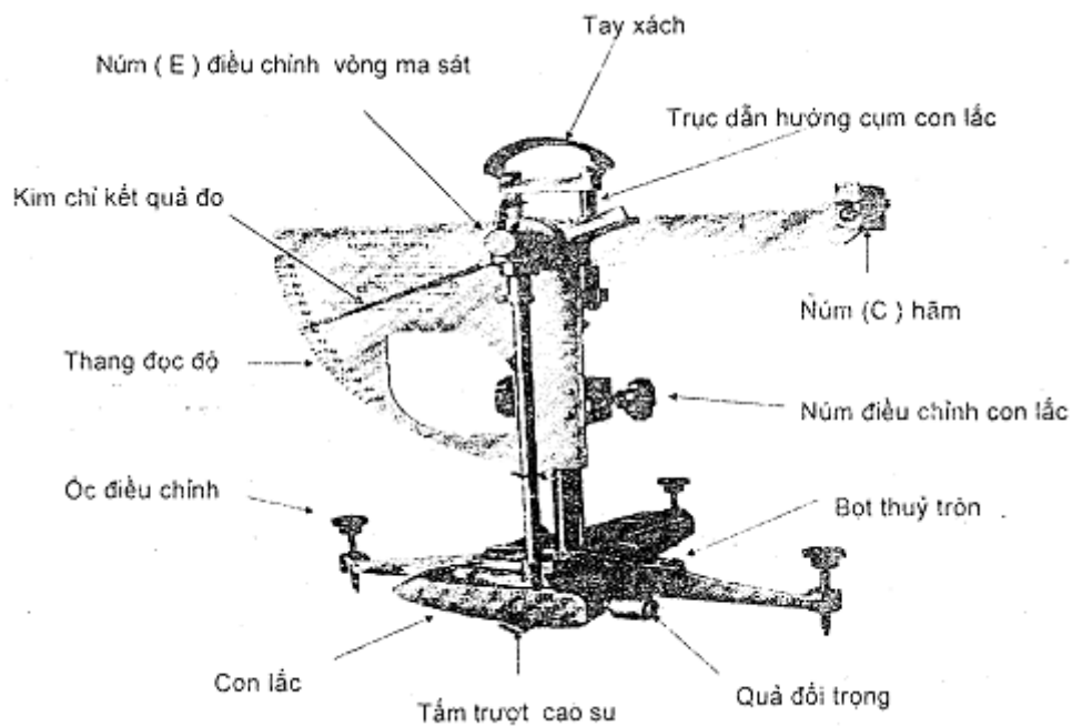
Hình 3 - Cấu tạo thiết bị con lắc nhám
